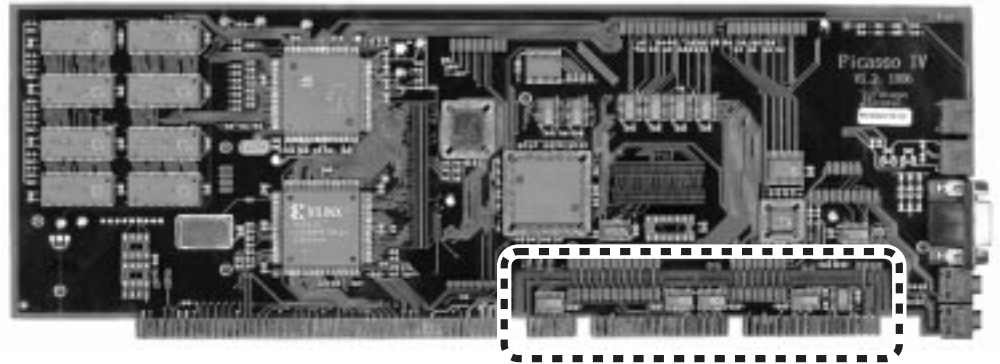
Abbildung 2: Die Videoplatine rechts unten
