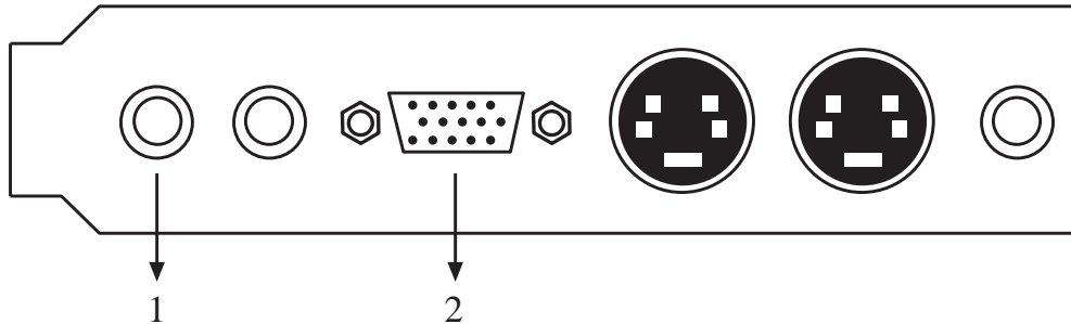
Abbildung 5: Ausgänge der Picasso IV
