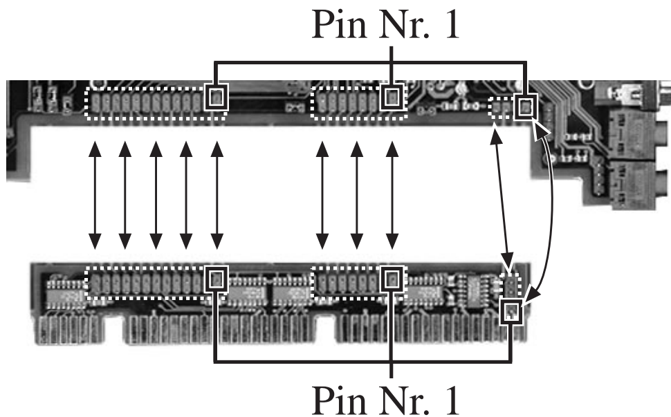
Abbildung 4: Verbinden der Platinen
